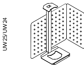
WSPORNIK POD KOMPUTER Z ZABUDOWĄ RASTROWĄ
